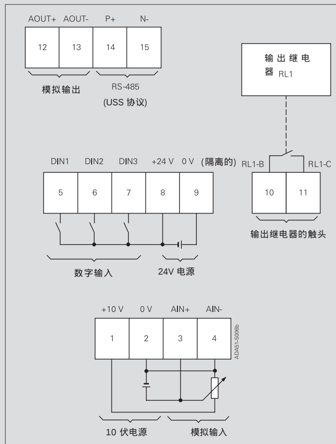
视图 A
